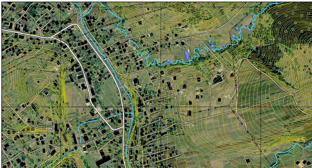
Рис.8. Фрагмент створеної ортофотокарти за матеріалами аерокосмічного знімання
