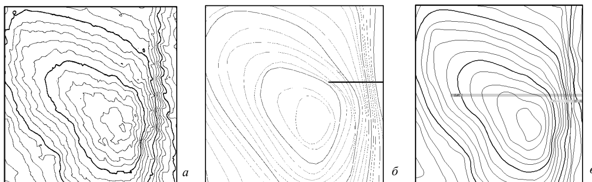
Рис.7. Фрагменти горизонталей, згенерованих в ГІС "Панорама"
