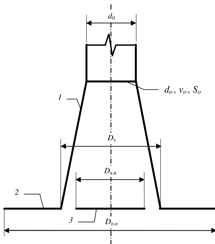
Рис.4. Схема конічного локального відсмоктувача: 1 – корпус відсмоктувача; 2 – повітрообмежник; 3 – центральна колова вставка
