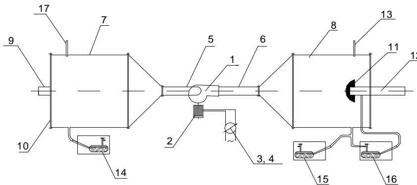
Рис. 3. Схема експериментального стенда: 1 – радіальний вентилятор; 2 – електродвигун постійного струму; 3 – автотрансформатор; 4 – випрямляч змінного струму; 5 – повітропровід на всмоктуванні; 6 – повітропровід на нагнітання; 7 – камера розрідження; 8 – камера плюсового надлишкового тиску; 9 – об’єкт досліджень – локальний відсмоктувач; 10 – знімна стінка; 11 – витратомірний колектор; 12 – вихідний патрубок; 13, 17 – термометри; 14, 15, 16 – різнищеві (диференційні) мікроманометри
