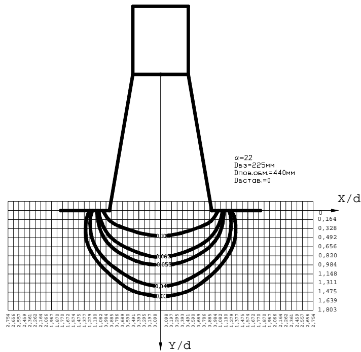
Рис. 5. Схема поля ізотах відсмоктуваного повітряного потоку
