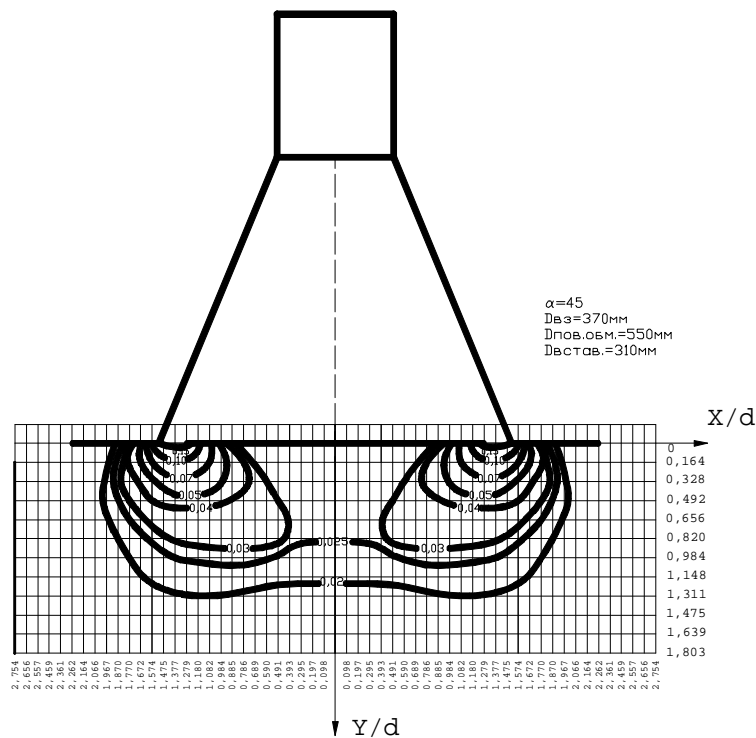
Рис. 8. Схема поля изотех відсмоктуваного повітряного потоку
