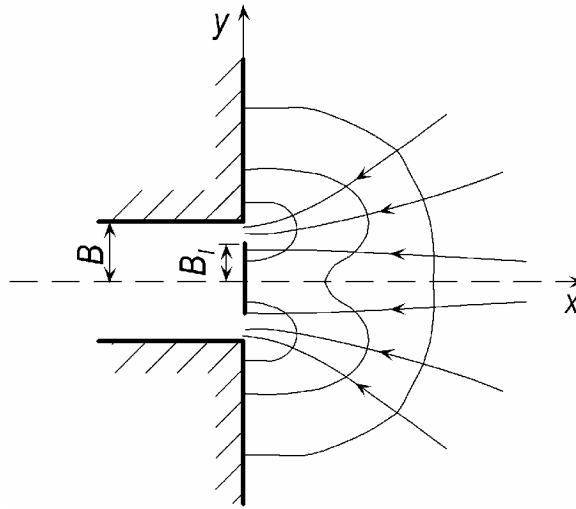
Рис.2. Схема стікання повітряного потоку в щілинний стіновий отвір, утворений за допомогою екрана
