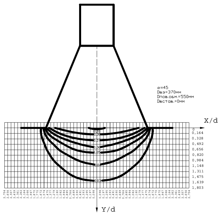
Рис. 7. Схема поля изотех відсмоктуваного повітряного потоку
