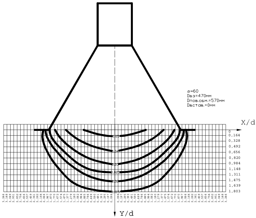
Рис. 9. Схема поля ізотах відсмоктуваного повітряного потоку
