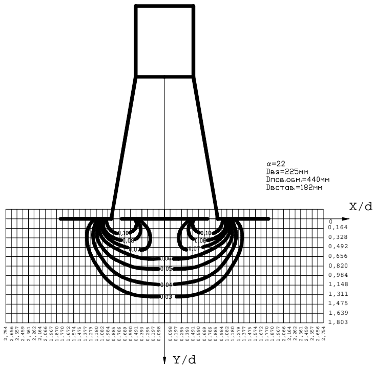
Рис. 6. Схема поля ізотах відсмоктуваного повітряного потоку
