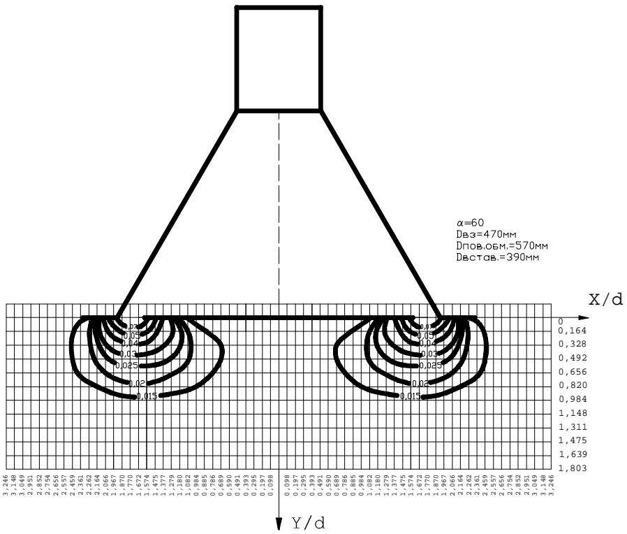
Рис. 10. Схема поля ізотах відсмоктуваного повітряного потоку
