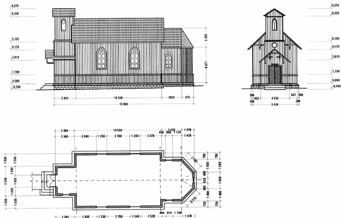
Рис. 2. Каплиця у с. Вовче. Обміри Мер'є О. 2003 р.
