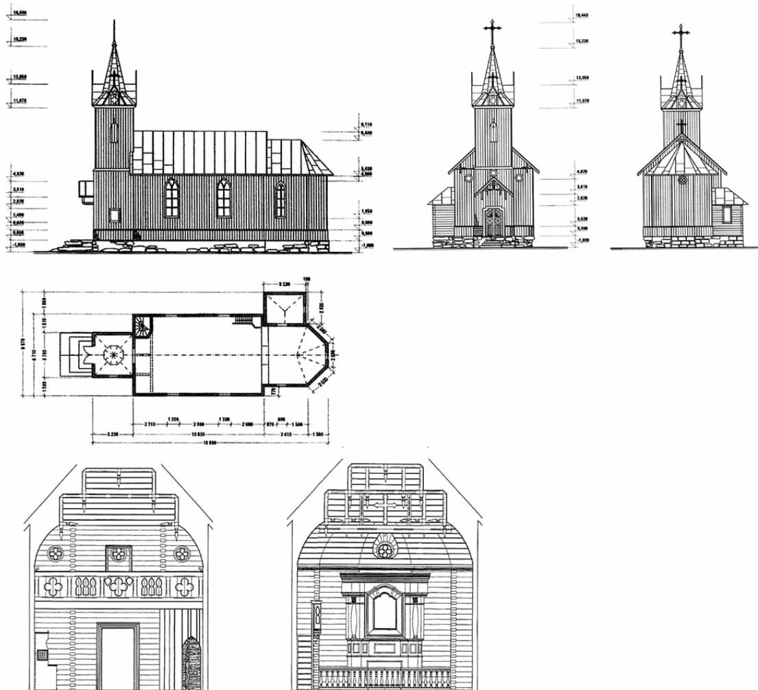
Рис. 4. Каплиця у Розлучі. Обміри Мер'є О. В. 2003 р.
